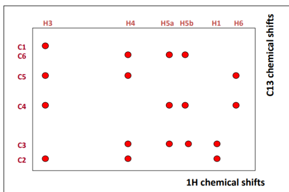
Figura 65: Rappresentazione ideale di uno spettro HMBC
